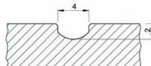
Schemat aplikacji frezowanej
