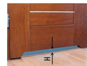
Podcięcie wentylacyjne H = 12 mm lub 30 mm
