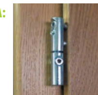
3 zawiasy dwuczopowe 3D z regulacją w trzech płaszczyznach (drzwi przylgowe) srebrne, w opcji za dopłatą osłonki - strony 51 - 52
