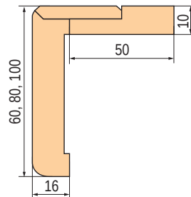
Opaska kątowna 60, 80, 100 mm z klipsem
