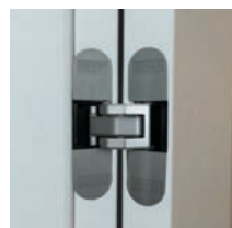
3 ukryte zawiasy regulowane srebrne, czarne, złote lub białe
