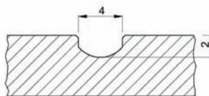
Schemat aplikacji frezowanej
