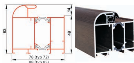
Ciepła ościeżnica aluminiowa z uszczelką do drzwi stalowych zewnętrznych 72 LUX, 72 LUX TERMO, 85 LUX TERMO PLUS
