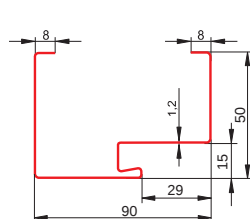
Ościeżnica stalowa z uszczelką do drzwi stalowych technicznych 40 FD-25/21B-40
