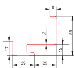
Ościeżnica stalowa z uszczelką do drzwi stalowych technicznych 40 FD-21/N
