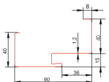
Ościeznica stalowa z uszczelką FD-25/21C
