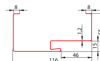
Ościeżnica stalowa z uszczelką do drzwi stalowych wewnętrznych 72 LUX FD-25/21B-72
