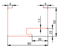
Ościeznica stalowa z uszczelką FD-25/21B
