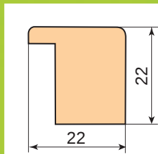
Listwa w standardzie
