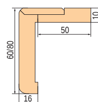
Opaska kątowna 60/80 mm z klipssem MDF za dopłatą
