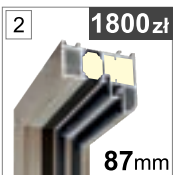
Ościeznica aluminiowa ALU/90 trzykomorowa z podwójnym uszczelnieniem z przegrodą PCW wypełnioną pianą
