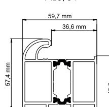
Profil ościeżnicy ALU/54
