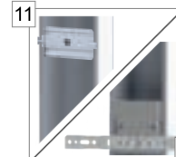
11 Elementy wzmacniające konstrukcję ościeżnicy z kotwami montażowymi lub bez 12. Ościeżnica 10/54, 11/54 12. Ościeżnica 15/54
